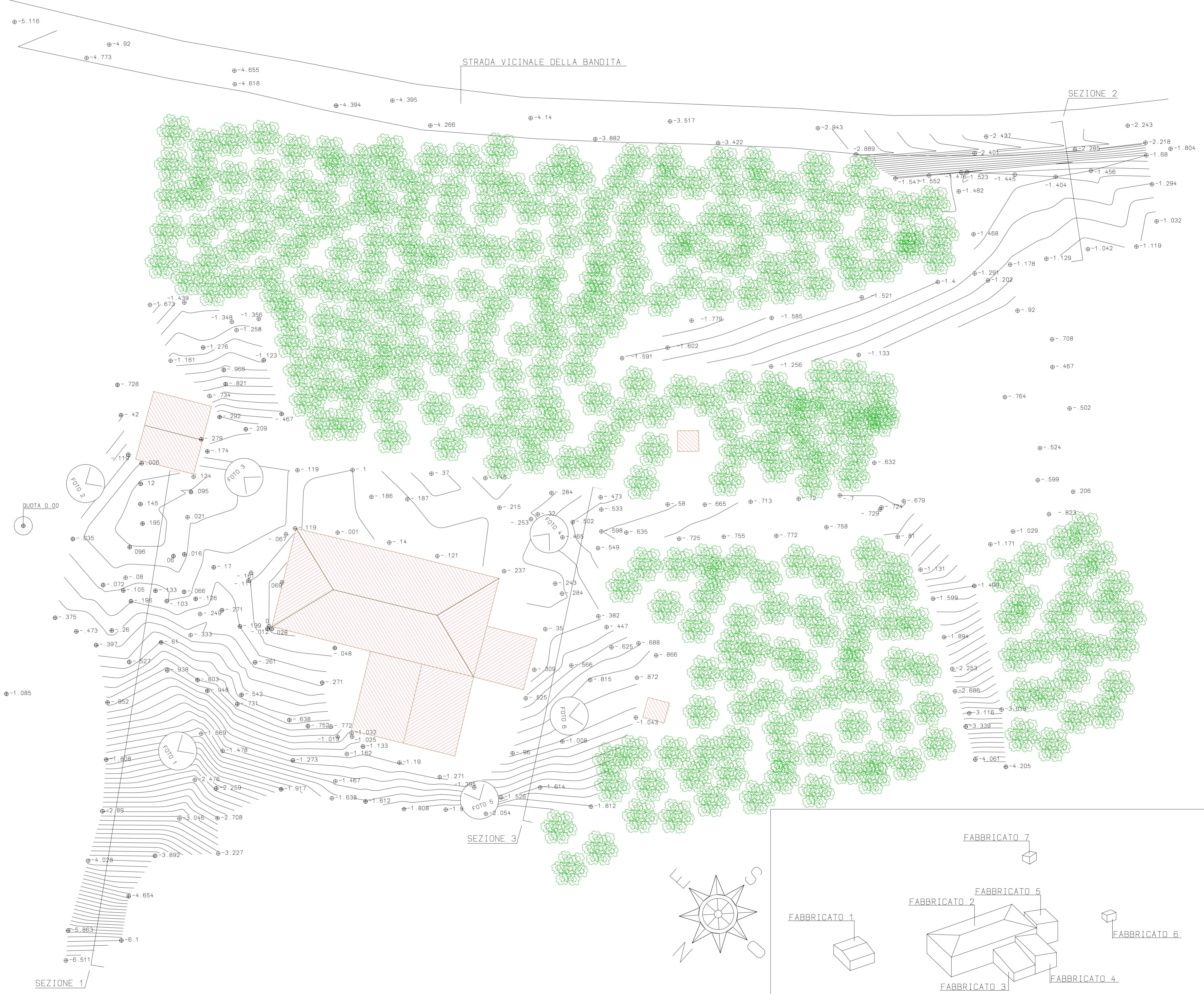
RILIEVO PLANOALTIMETRICO SCALA 1:200
